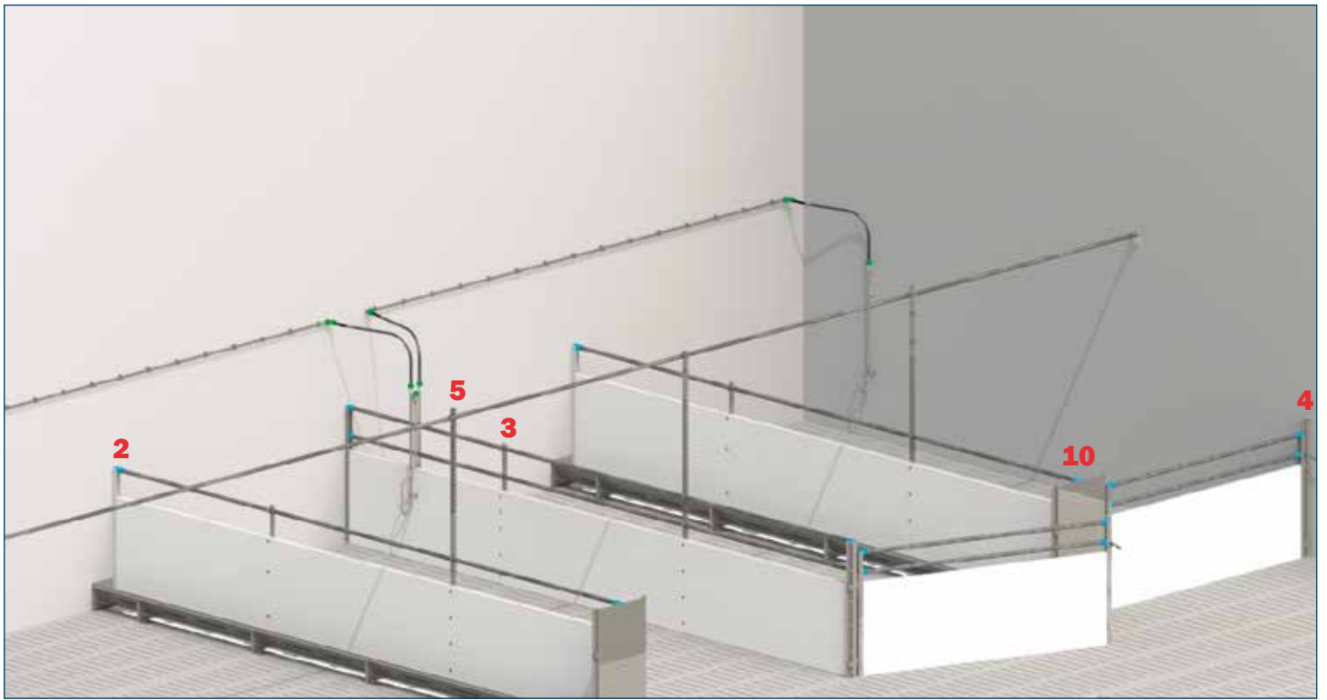
Mastbucht für Flüssigfütterung mit Edelstahl-Doppeltrog und Edelstahl-Kopfplatte (Koteinwurfschlitz unter dem Trog). Trennwandbeschläge Typ 3 mit Schwenktorbeschlägen 1,00 m hoch. Ein Profilstützpfeiler (3) ist durch einen V2A-Winkelpfeiler (5) mit Stabilisationsrohr ersetzt worden.
