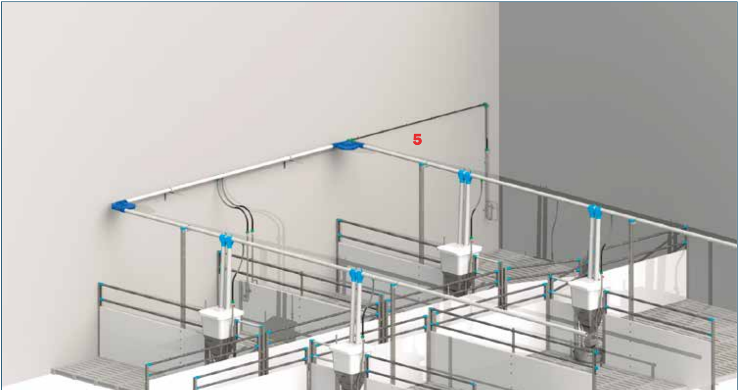
Mastbucht mit Stichgang fr Trockenftterung mit Trennwandbeschlge Typ 2, Schwenktorbeschlge, V2A-Winkelpfosten (5), Wasserarmaturen und Mastautomat S-Flex.
