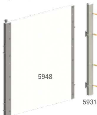
Drehtorbeschlag 1,00 m hoch
