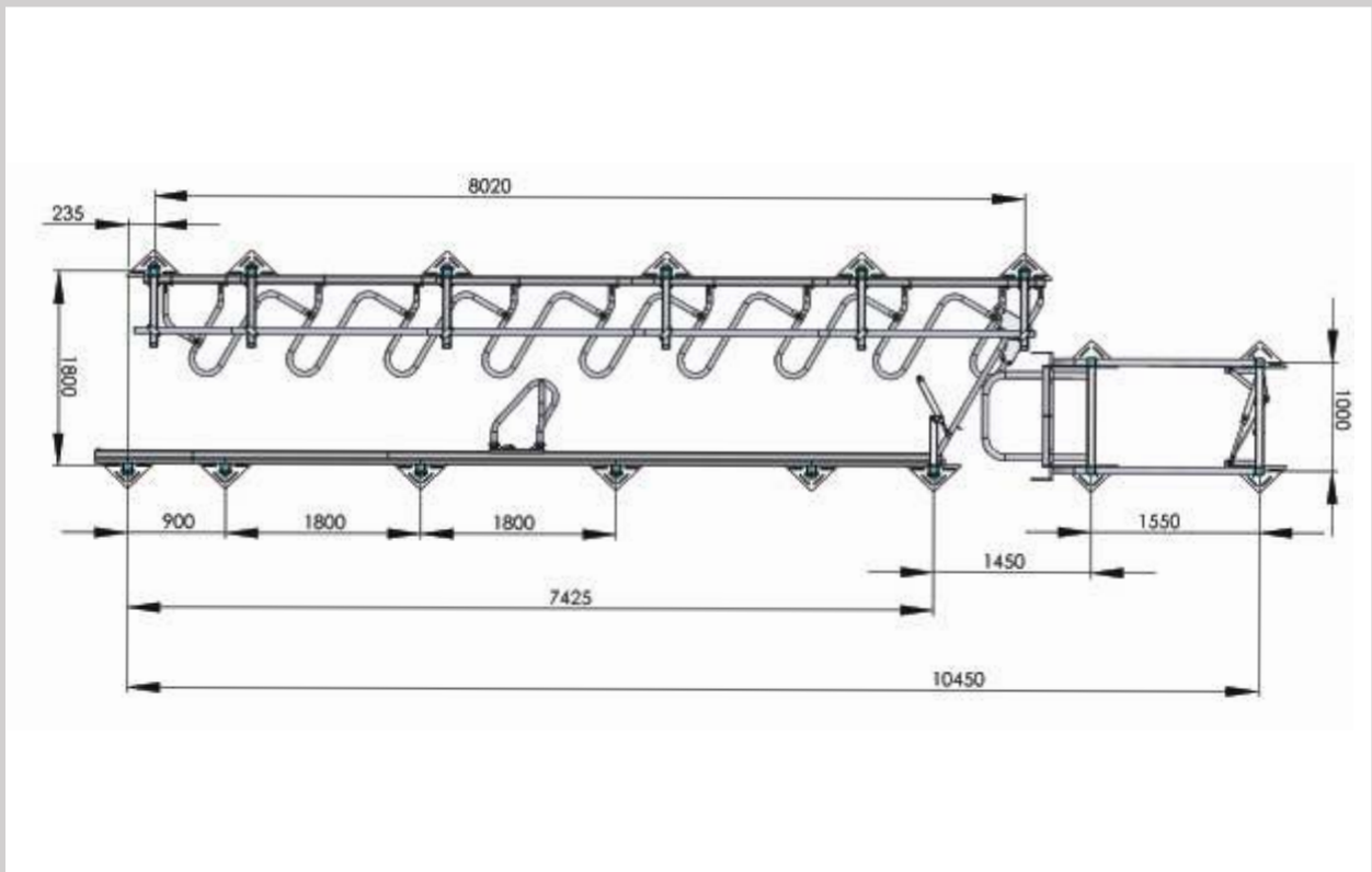
Behandlungsstraße mit Einzelbehandlungstand 8 Kuhplätze
